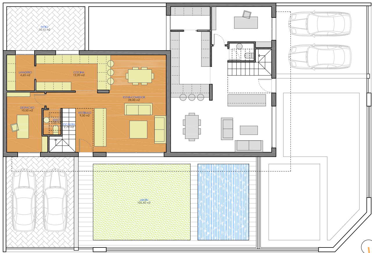
PLANTA BAJA
